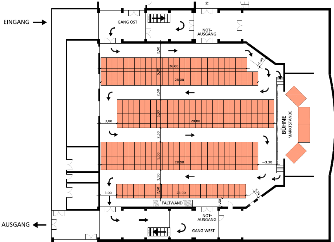
HALLENPLAN 1. UNTERGESCHOSS
