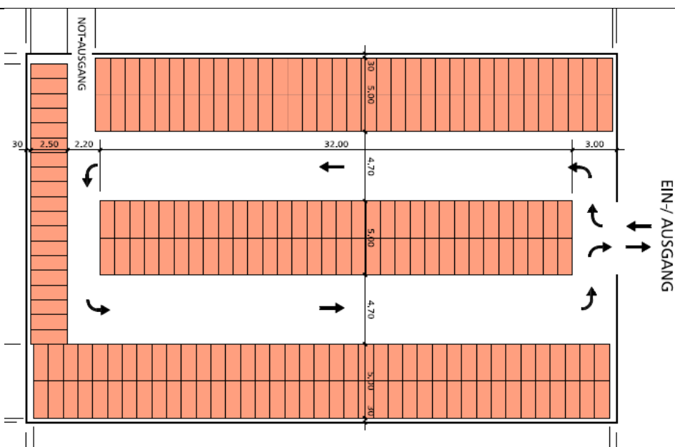
AUSSTELLERZELT 25.00 x 40.00 m
